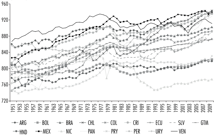
Gráfica 3. Logaritmo natural del PIB per cápita anual de los (17) países de América Latina: 1951-2010 (multiplicado por 100)
